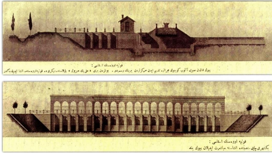
Şekil 3. Bendin Osmanlı Dönemindeki İlk Proje Çalışmaları (Yılmaz, 2010: 11)
