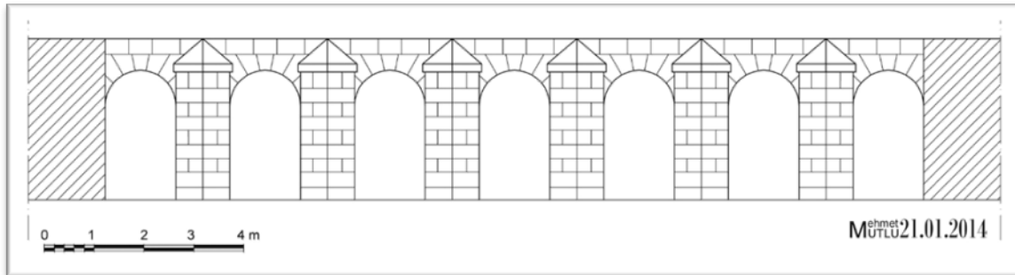
Ana Kanal Bağlantısı Memba Cephesi
