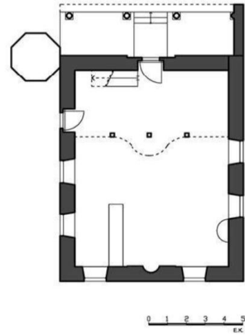
Görsel 5. Ortaköy Camii Planı
